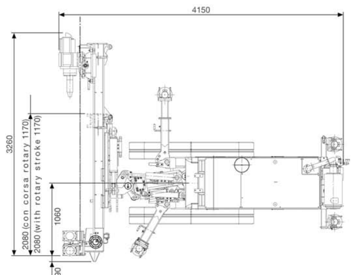
Disegno 4 / Drawing 4 Esecuzioni di tiranti / Anchor execution
