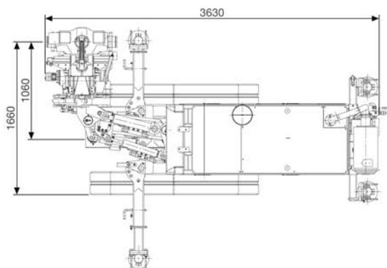
Disegno 3 / Drawing 3 Perforazioni verticali in prossimità di pareti / Drilling near vertical walls
